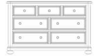
3 OVER 4 CHEST H: 841 W: 1356 D: 514
