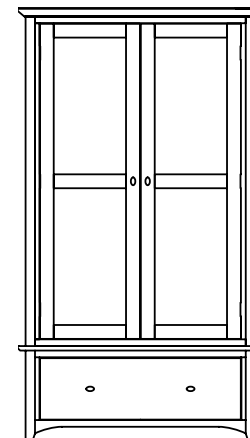
1 DRAWER WARDROBE H: 1910 W: 1095 D: 580
