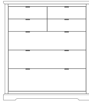
2 + 2 CHEST H: 980 W: 900 D: 450
