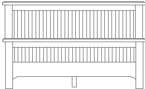
4 1/6" HIGH FOOT END BED H: 1015 W: 1522 D: 2130
