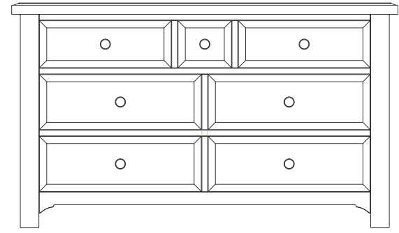
3 OVER 4 CHEST H: 785 W: 1346 D: 430
