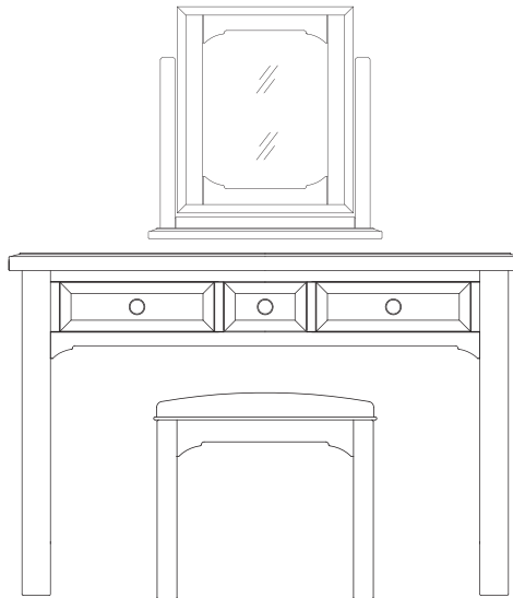
DRESSING TABLE H: 780 W: 1170 D: 430
