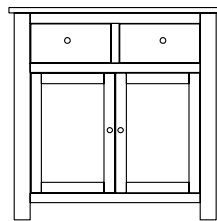
SIDEBOARD H: 800 W: 800 D: 340
