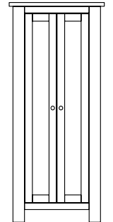
2 DOOR CUPBOARD H: 1150 W: 500 D: 300
